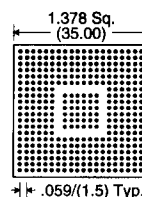
Footprint 372
