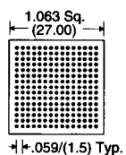
Footprint 225
