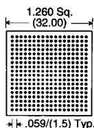
Footprint 324-3
